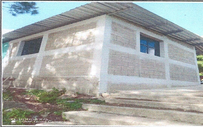
Foto 1: Area lateral donde se realizo el mejoramiento de la estructura tipo portico para la cocina, instalación de techo y ventanas.
