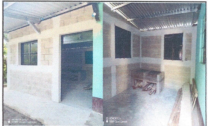
Foto 2: Area frontal, donde se realizo el mejoramiento la estructura tipo portico para la cocina, con paredes de concreto, losa de piso de concreto, techo de lamina, ventanas, puerta y polleton.
